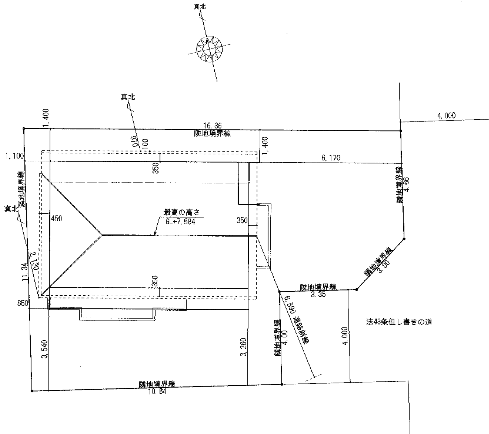
配置図 S:1/100
